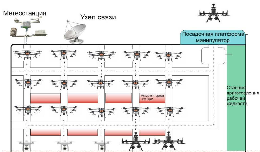
Рис. 3. Схема прототипа дронопорта*
