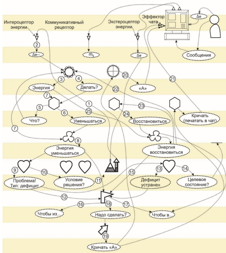
Рис. 1. Базовая мультиагентная нейрокогнитивная архитектура интеллектуального агента
