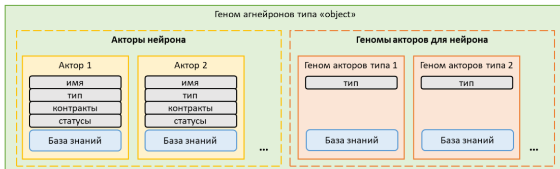
Рис. 5. Схема строения генома агнейрона
