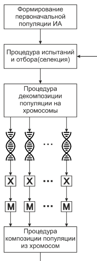
Рис. 6. Многохромосомный алгоритм обмена генетическими данными интеллектуальных агентов: X – операция кроссинговера, M – операция мутации
